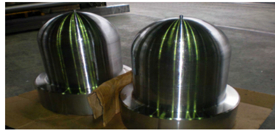
L600、 \phi 500 の加工
