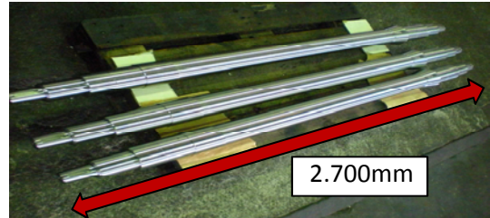
ステンレスの長尺シャフト加工
