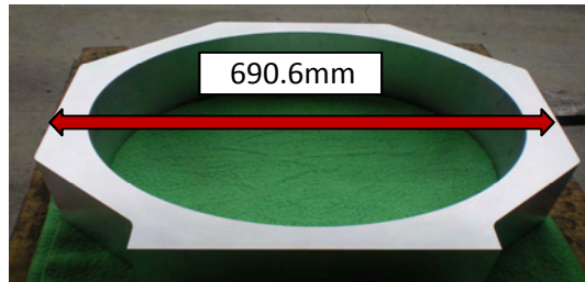
アルミ半導体ケースの加工
