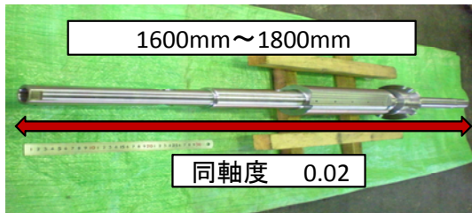
SCM長尺シャフト加工
