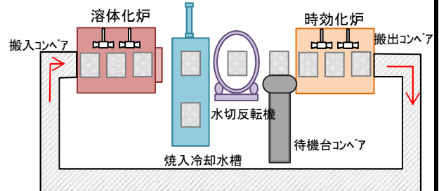
社内の連続式大型熱処理炉の工程(T6処理)
