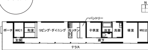
平面図
