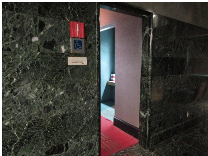
○南側多目的トイレ（最小通行幅 80cm）
