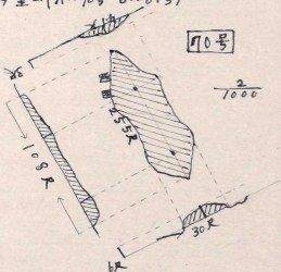
大所川東北競馬場展望(A=70号 B=69号)
