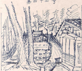
進藤初太郎氏宅裏屋敷柏荷ヲ祀ル第44号古墳
