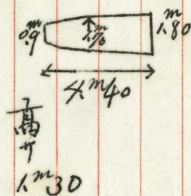
石槨 平面
