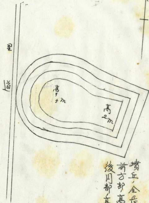
荒砥 三五五號古墳平面圖
