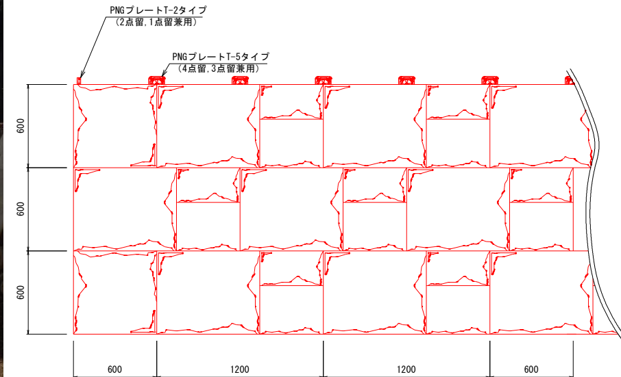
もたれ式擁壁正面図
