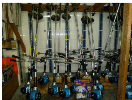
貸出し用の森林整備作業器具
