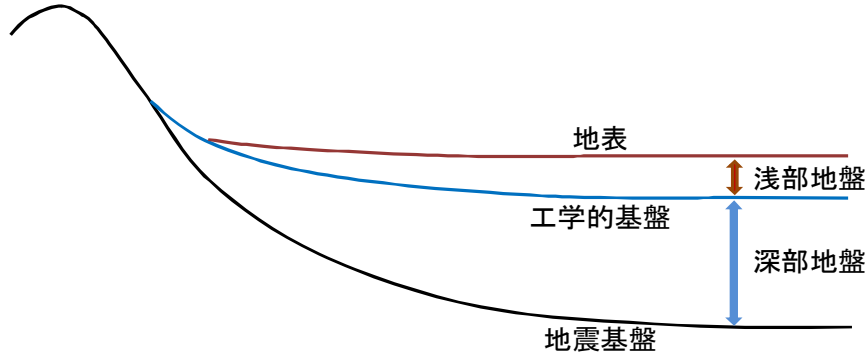
図 4.1 地盤構造の模式断面図
