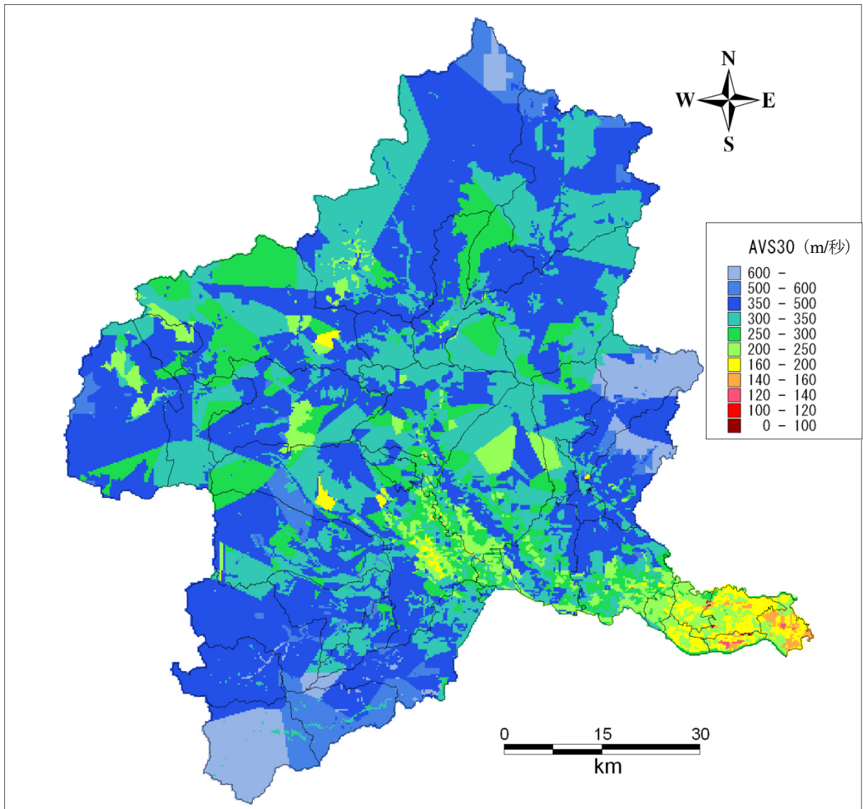
図 4.8 作成した地盤モデルの AVS30 の分布
