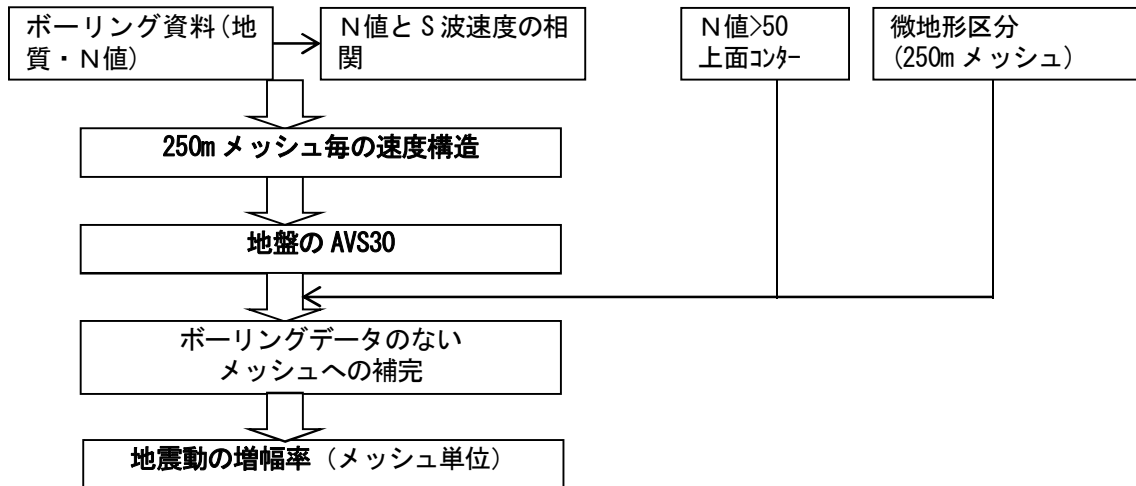
図 4.3 浅部地盤構造モデルの作成フロー
