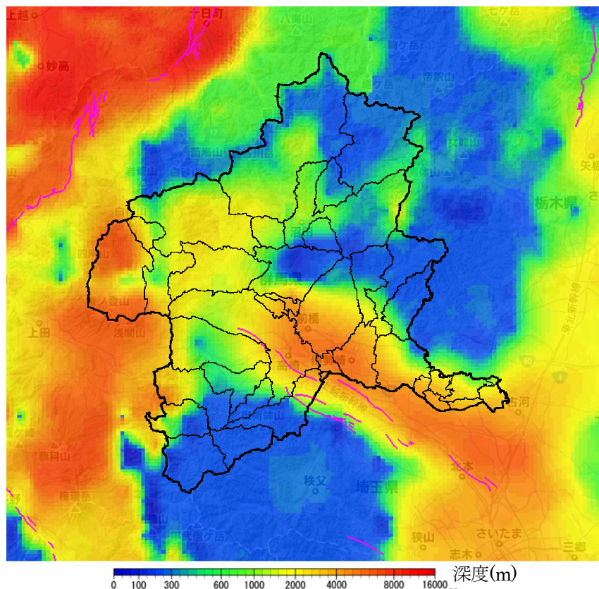
図 4.2 深部地盤モデルにおける地震基盤の上面深度分布図 (J-SHIS より：行政界を加筆)
