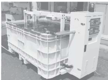
①コンニャク種芋温湯消毒装置
