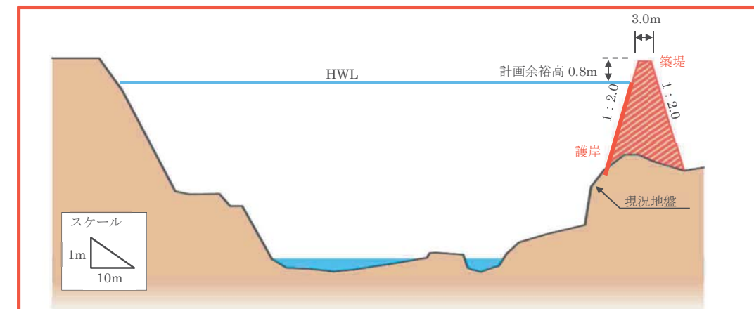
図 4.25 代表横断面図（赤谷川：⑧日和橋下流）
