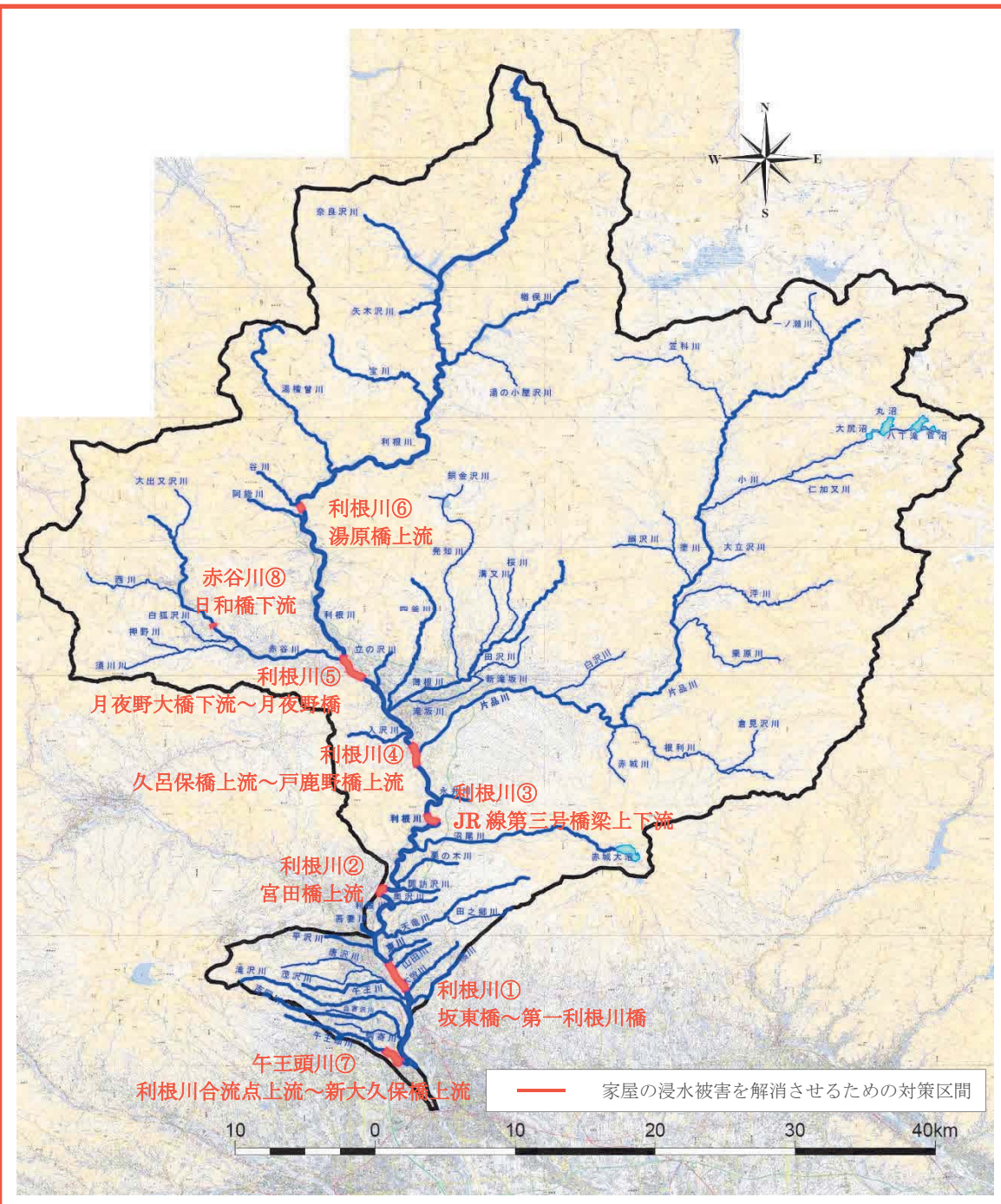
図 4. 1 整備対象区間位置図
