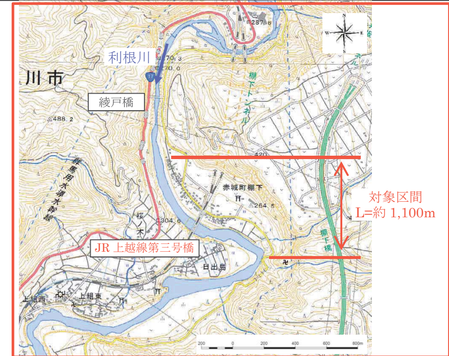
図 4. 10 位置図（利根川：③JR 上越線第三号橋梁上下流）
