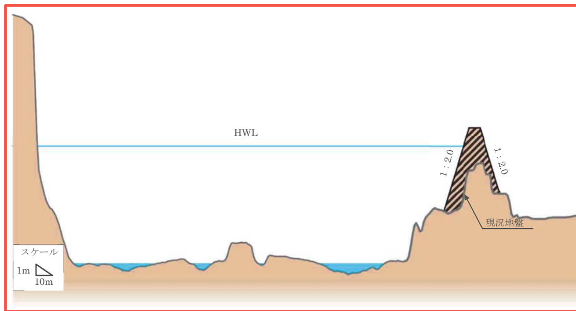
図 4. 3 代表横断面図（利根川：①坂東橋～第一利根川橋）
