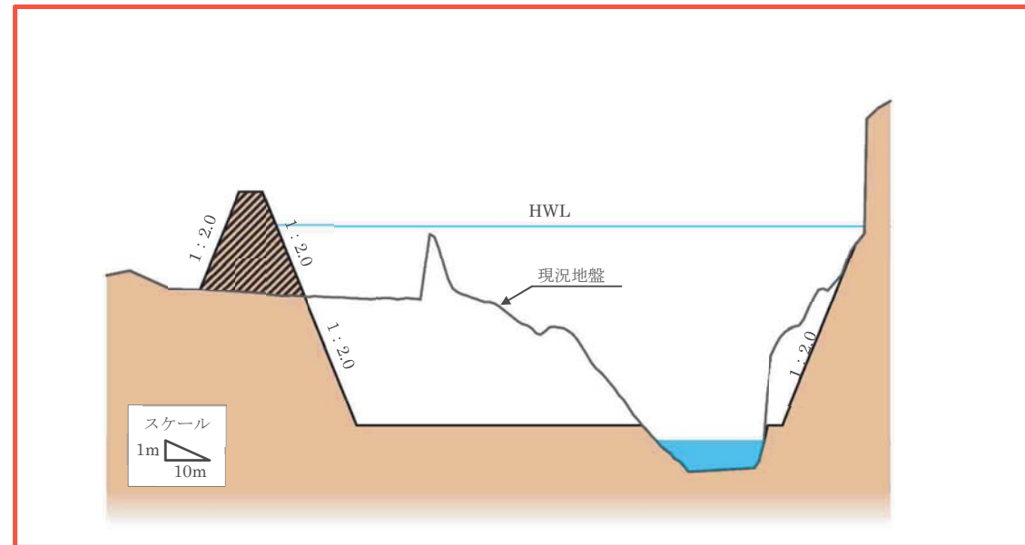
図 4.6 代表横断面図（利根川：②宮田橋上流）
