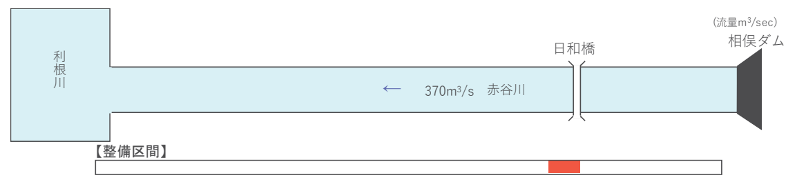
図 4.26 流量配分図（赤谷川）
