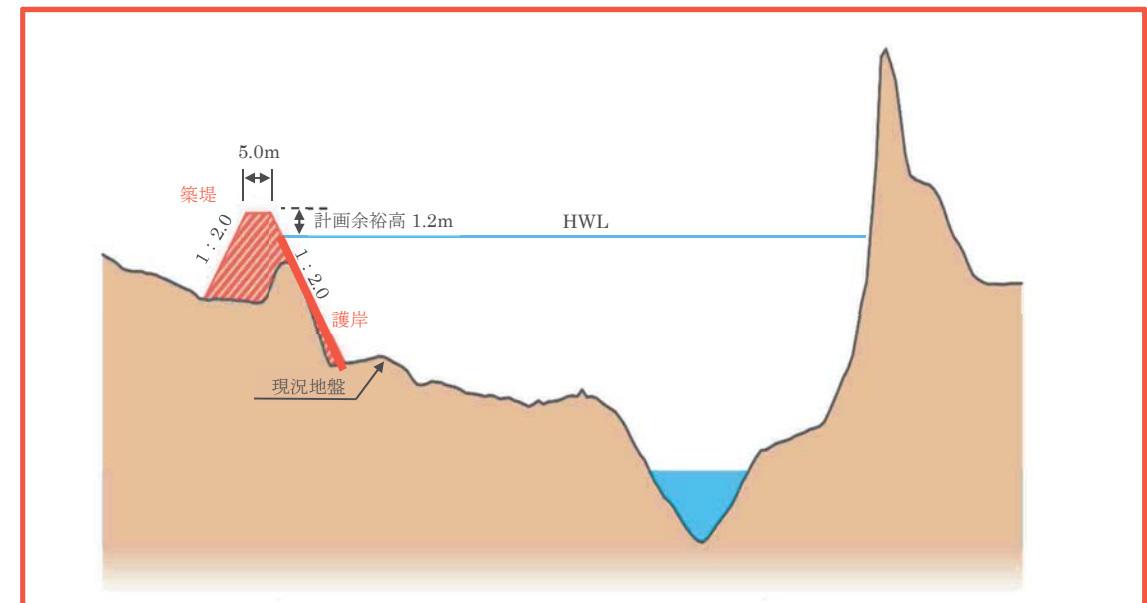
図 4.9 代表横断面図（利根川：③JR 上越線第三号橋梁上下流）
