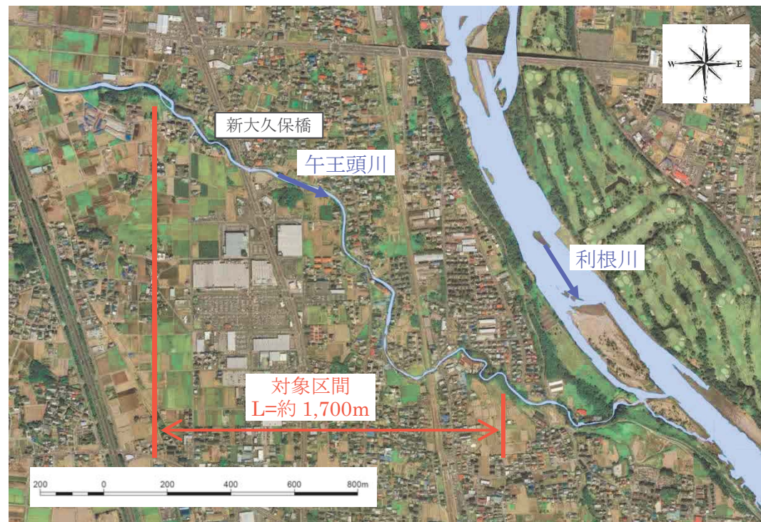
図4.24 航空写真（午王頭川：⑦利根川合流点上流～新大久保橋上流）
