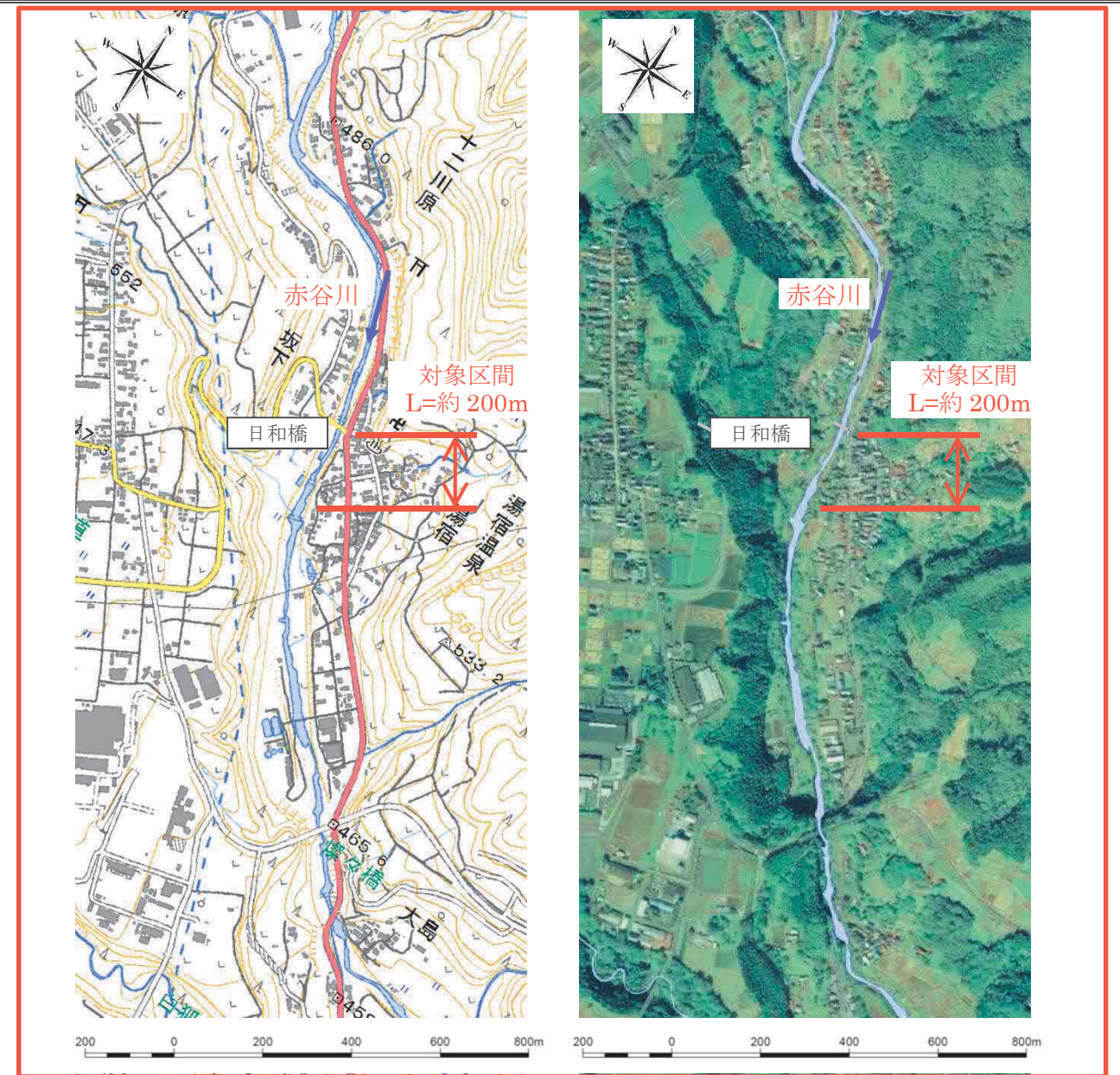
図4.27 位置図（赤谷川：⑧日和橋下流） 図4.28 航空写真（赤谷川：⑧日和橋下流）
