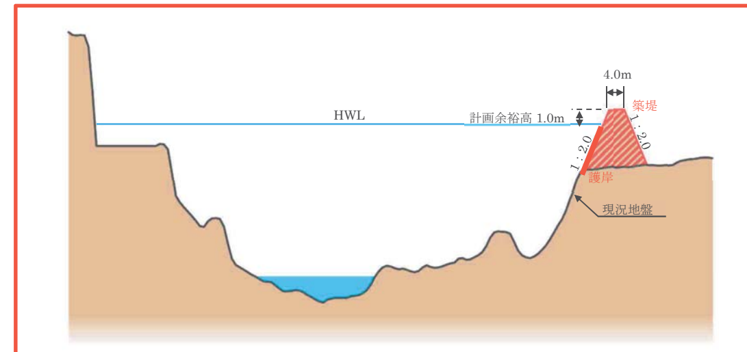
図 4.18 代表横断面図（利根川：⑥湯原橋上流）
