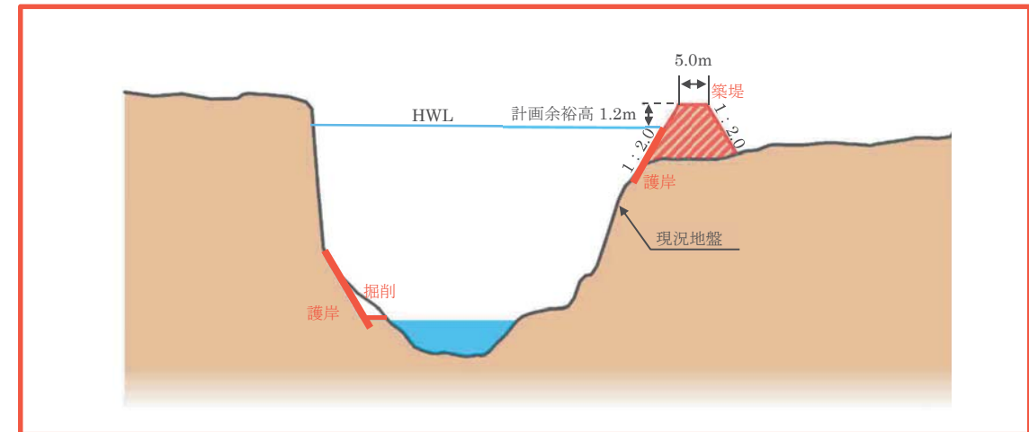
図 4.12 代表横断面図（利根川：④久呂保橋上流～戸鹿野橋上流）
