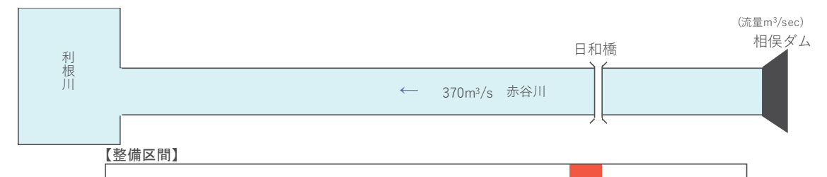
図 4.26 流量配分図（赤谷川）
