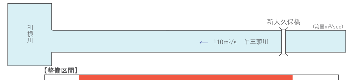
図 4.2.2 流量配分図（午王頭川）
