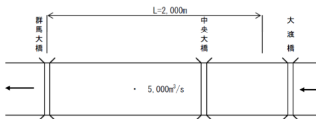
計画流量配分図
