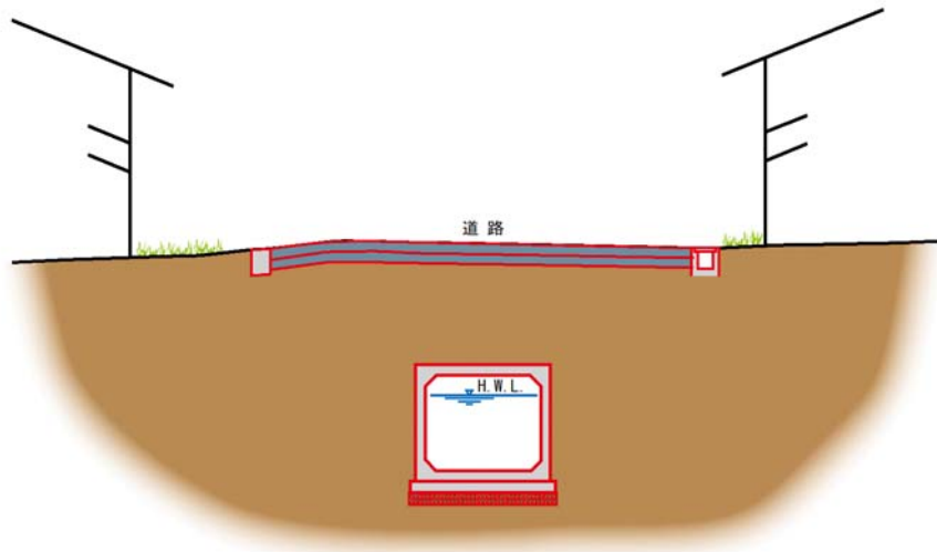
図 4.6 治郎兵衛川代表断面図（地下放水路）
