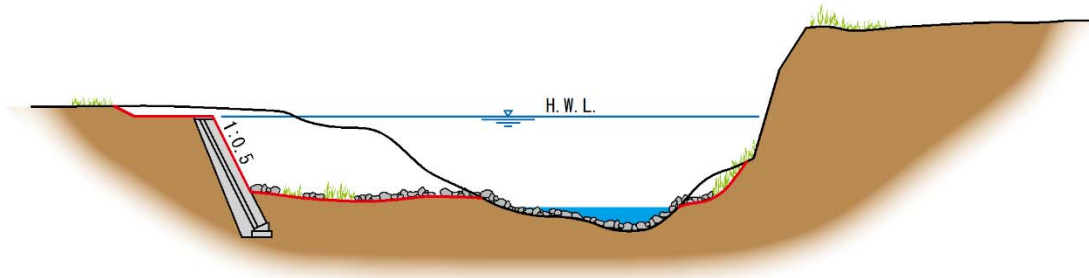
図 4.2 名久田川代表横断面図
