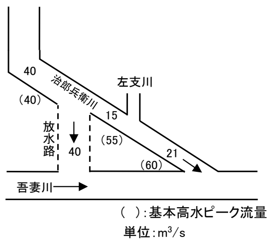
図 4.7 治郎兵衛川計画流量配分図
