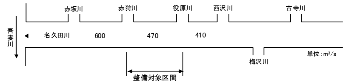
図 4.3 名久田川計画流量配分図
