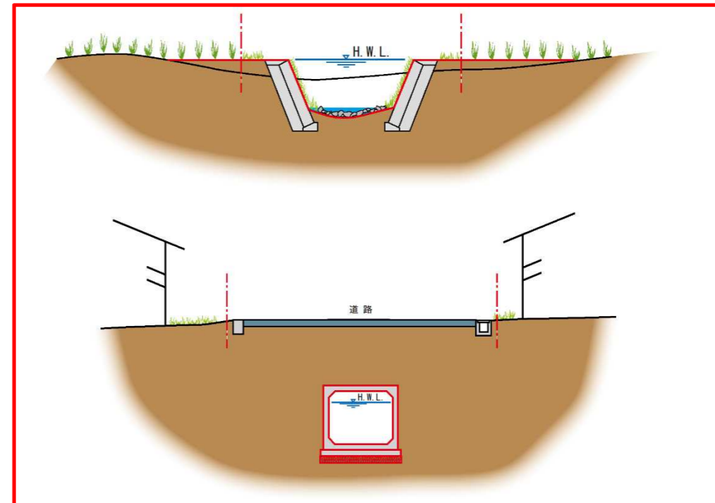
図 4.6 治郎兵衛川代表断面図（上：開水路、下：暗渠）
