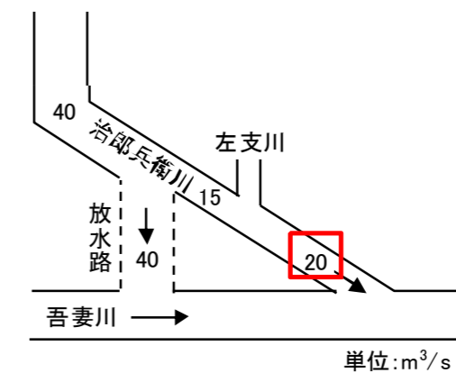
図 4.7 治郎兵衛川計画流量配分図
