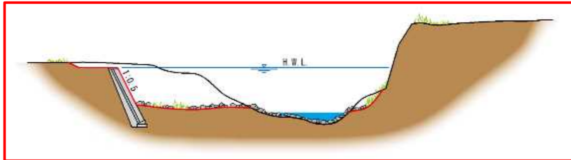
図 4.2 名久田川代表横断面図
