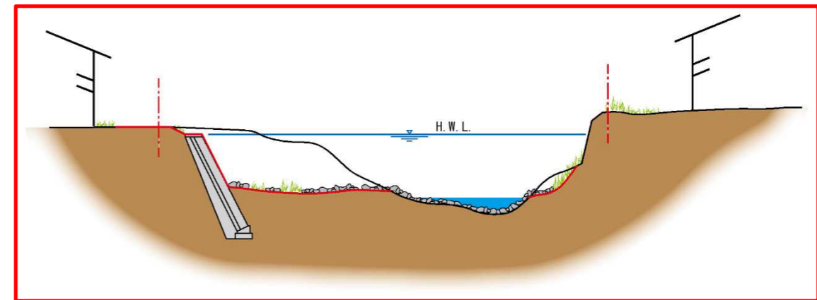
図 4.2 名久田川代表横断面図
