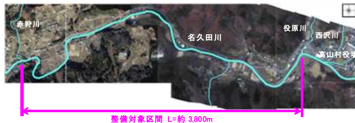
図 4.5 名久田川整備位置図
