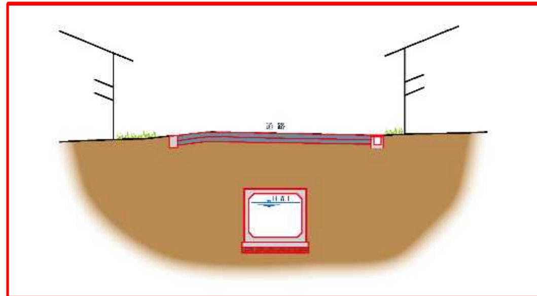
図 4.6 治郎兵衛川代表断面図（地下放水路）
