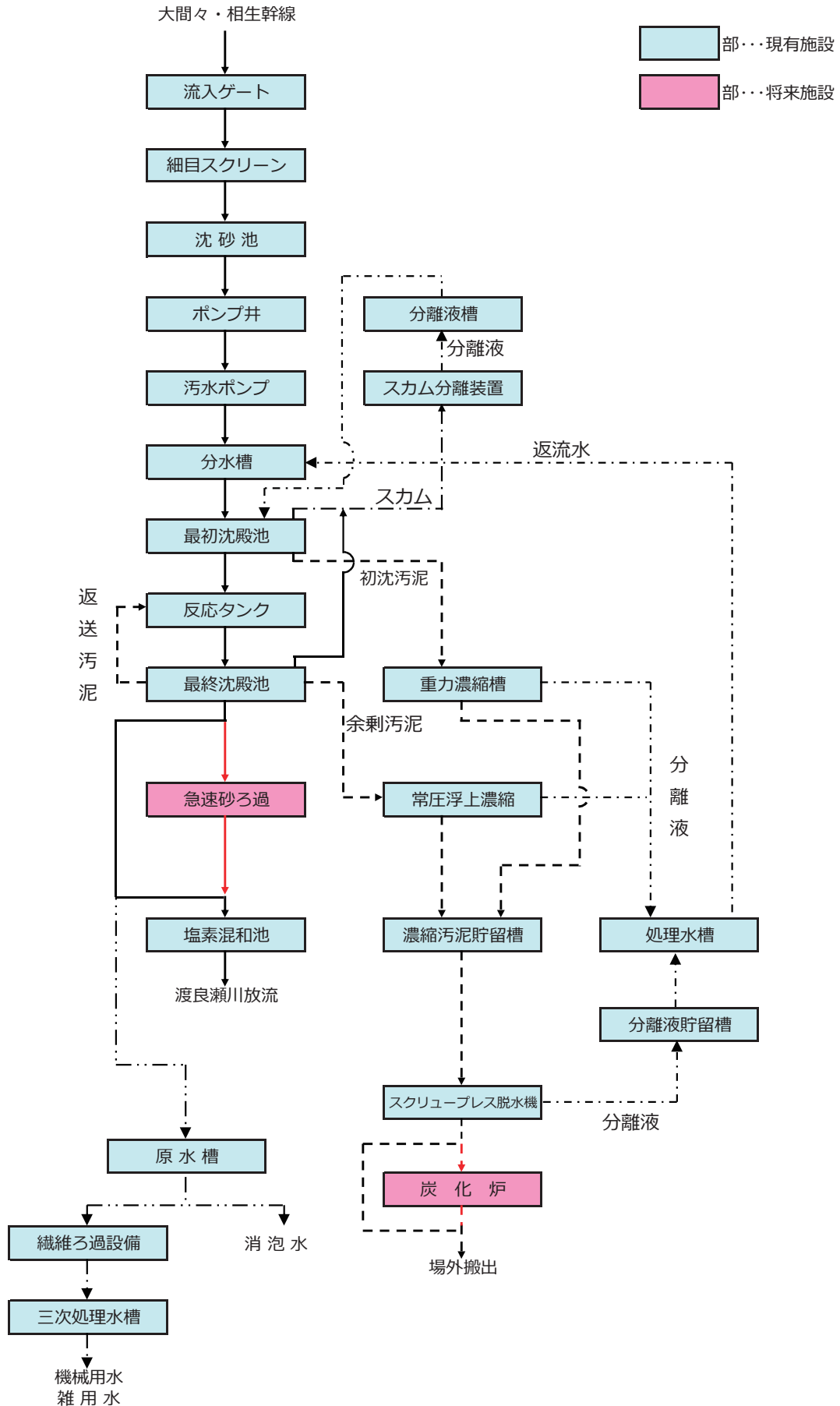
(4) 処理系統図
