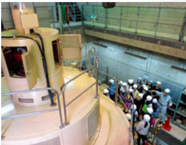
水車発電機を見学する様子（奈良俣発電所）
