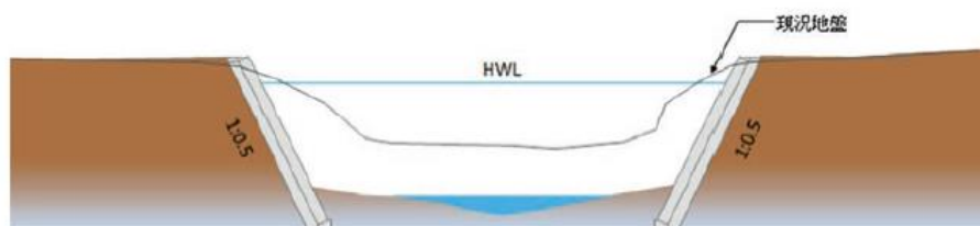
図 4-3 代表横断図（休泊川）
