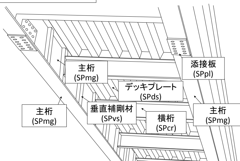
上部構造-デッキプレート形式②
