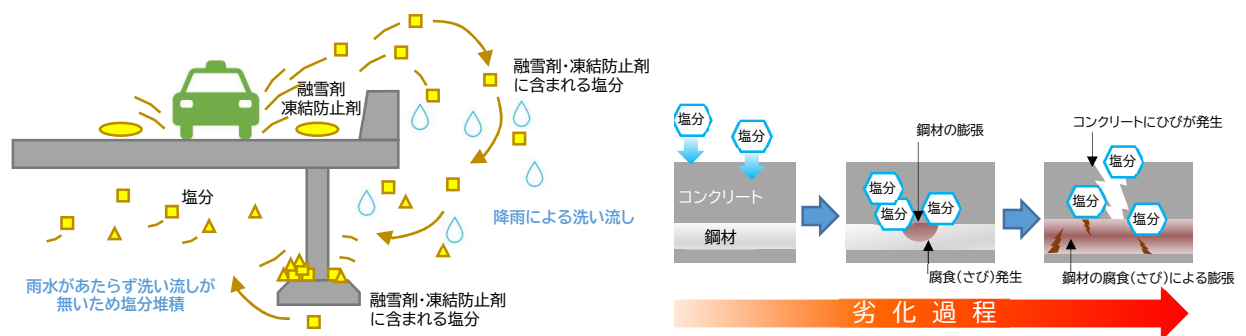
図 1-14 凍結防止剤による劣化と塩害メカニズム
