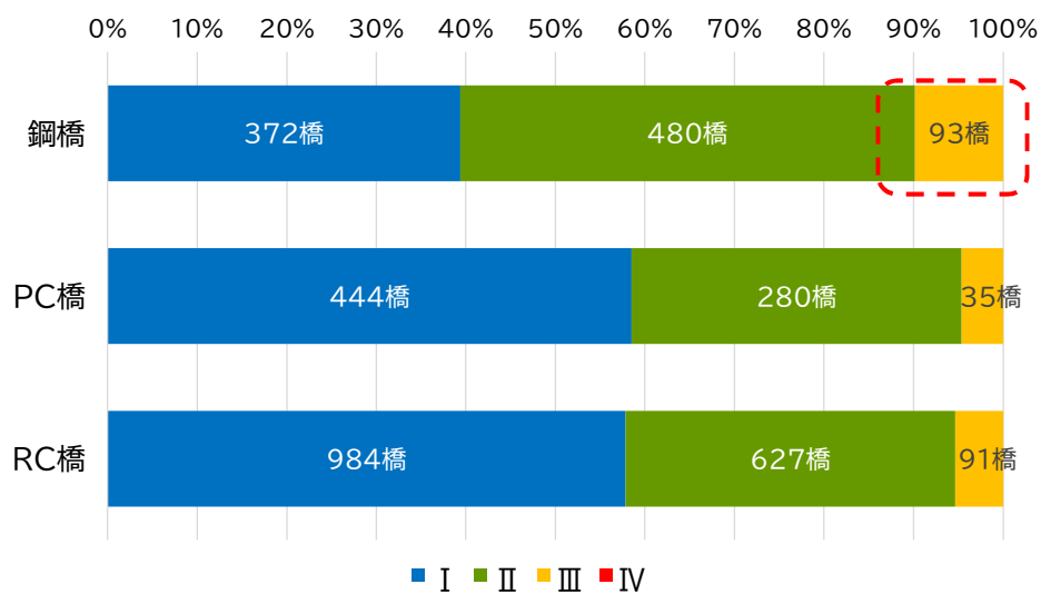
図 1-12 上部工使用材料別の健全性(2巡目点検)
