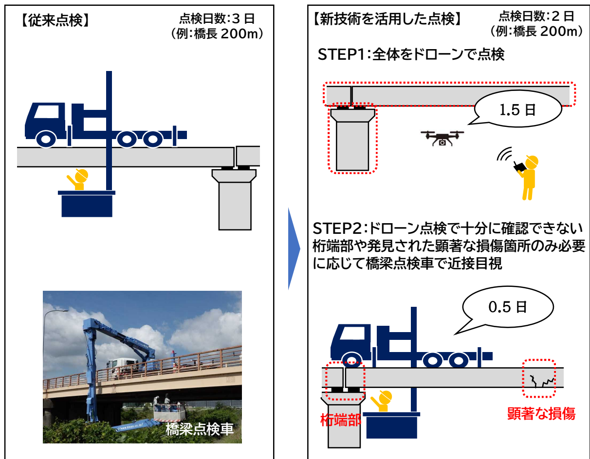
図 2-1 従来点検と新技術(ドローン)を活用した点検の比較
