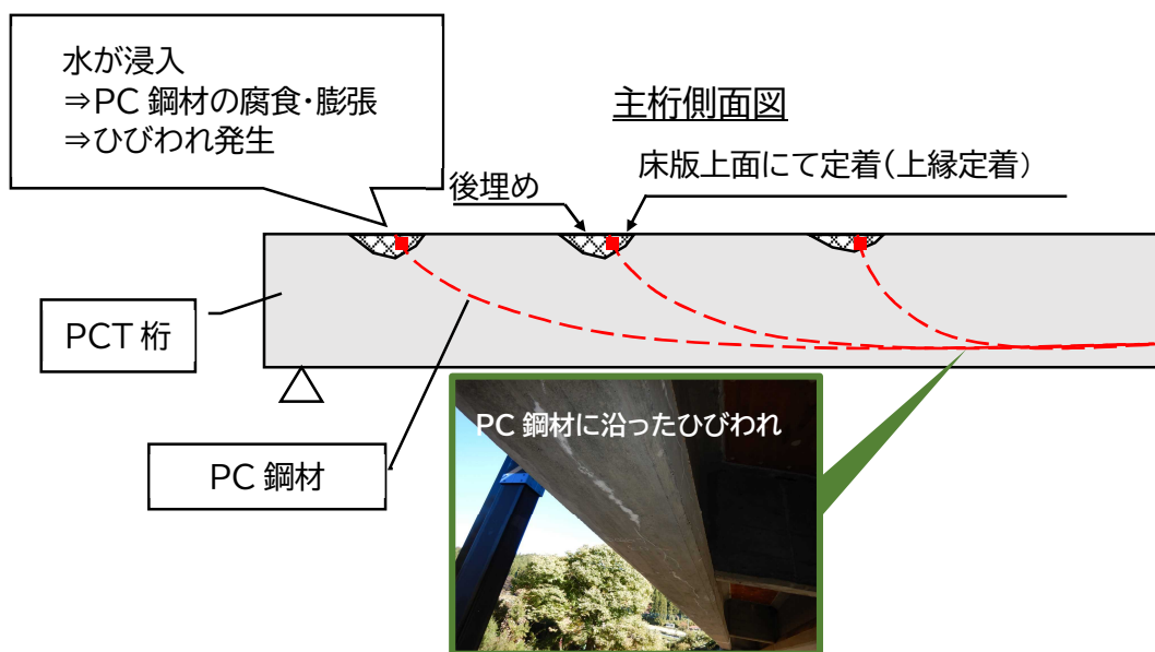
図 1-21 PC 橋に発生している健全性Ⅲの損傷傾向
