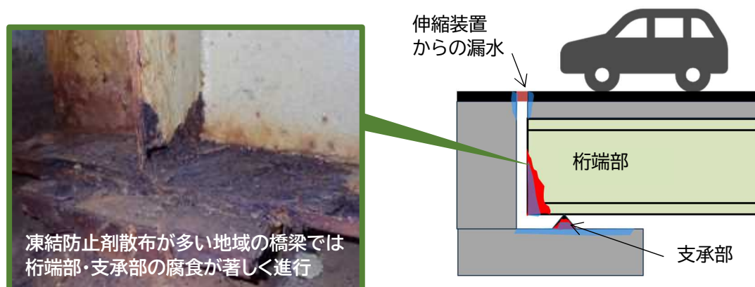
図 1-16 桁端部・支承部の腐食事例
