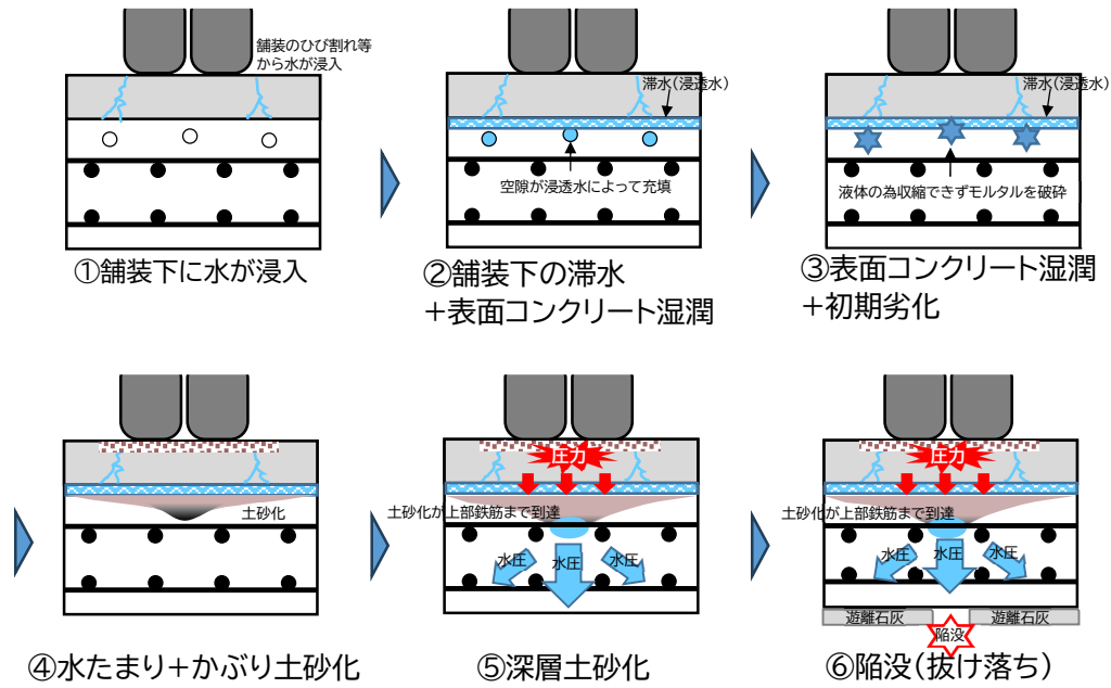
図 1-20 床版の土砂化(輪荷重による)メカニズムイメージ
