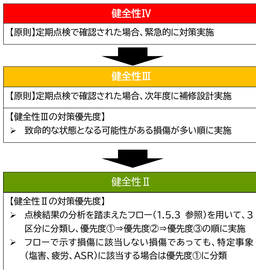
図 1-22 対策の優先順位の考え方
