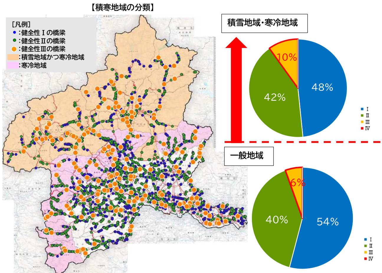
図 1-13 群馬県内積寒地域の分類及び健全性の分布
