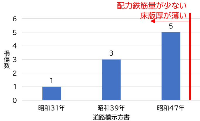
図 1-17 鋼橋(RC 床版)に発生している健全性Ⅲの損傷傾向
