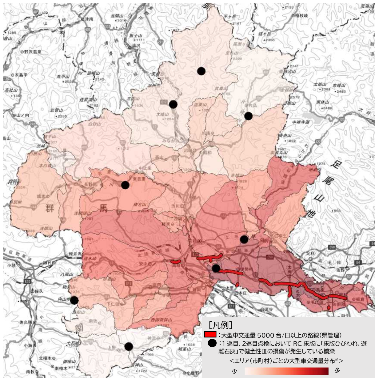
図 1-19 RC 床版に健全性Ⅲの損傷が発生している橋梁の位置図と大型車交通量
