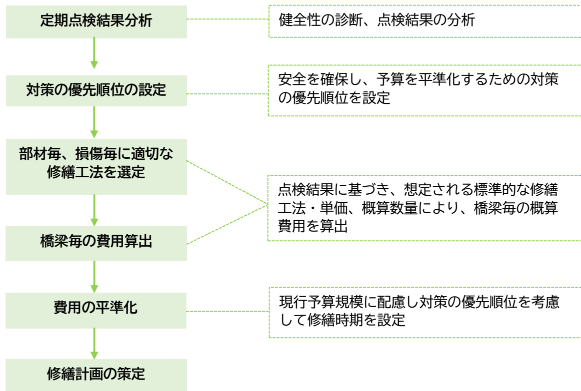
図 1-3 修繕計画策定フロー
