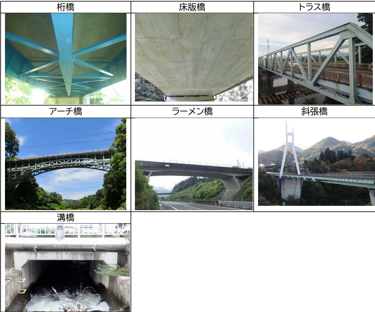
写真 1-2 上部工構造形式例
