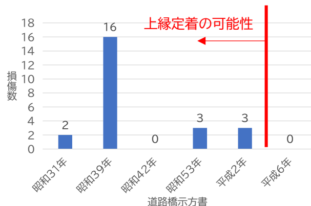
【PCT 桁にひびわれが発生している橋梁の設計基準】
