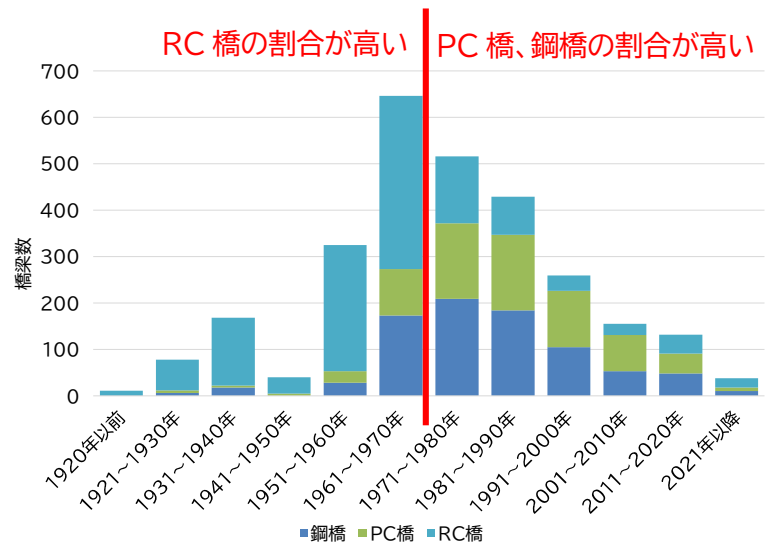
図 1-7 架設年度(10 年単位)毎の上部工使用材料別橋梁
