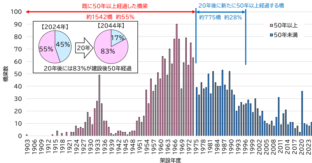
図 1-1 架設年度別橋梁数
