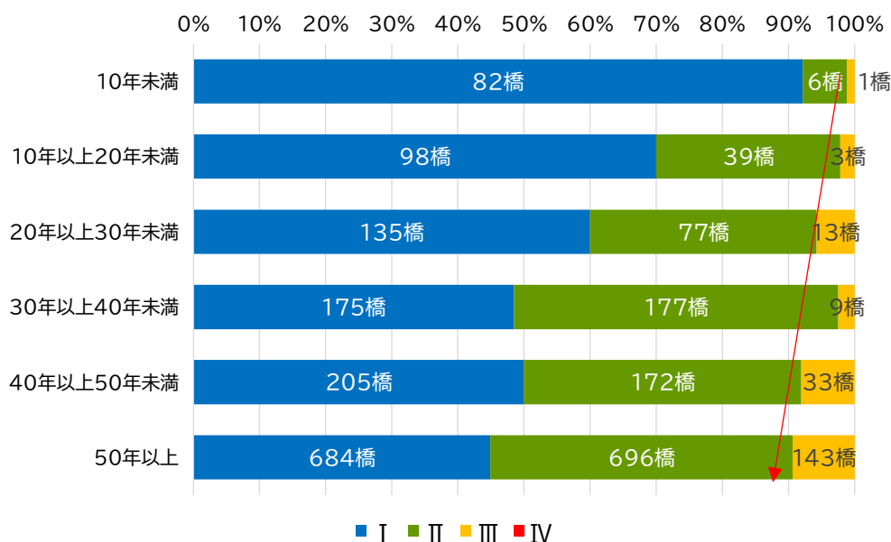
図 1-10 建設後経過年数別の健全性(2巡目点検)
