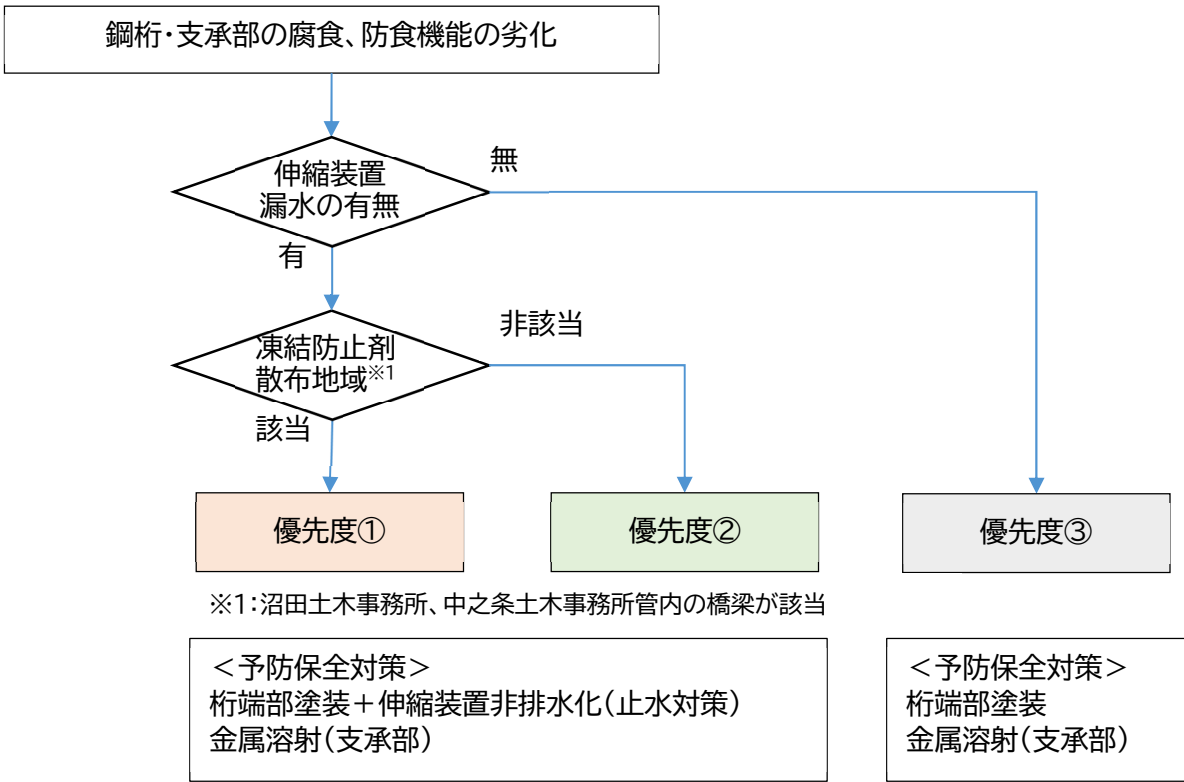
図 1-23 健全性Ⅱの優先度評価フロー(鋼桁・支承部の腐食、防食機能の劣化)
