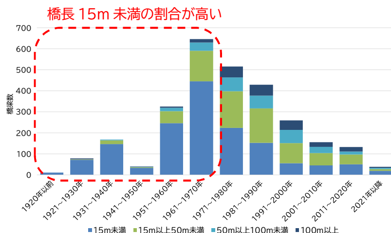
図 1-5 架設年度(10 年単位)毎の橋長区分別橋梁数
