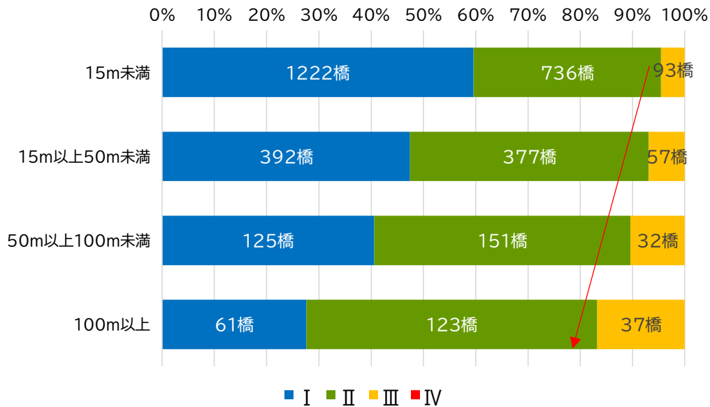
図 1-11 橋長区分別の健全性(2巡目点検)
