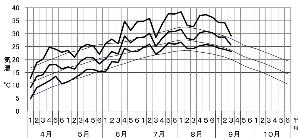
図1 気温
