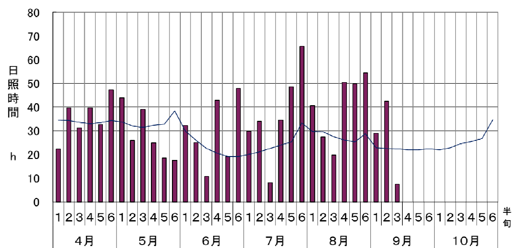
図3 日照時間
