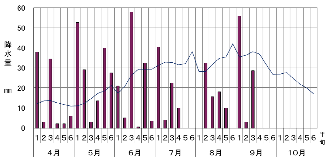
図2 降水量
