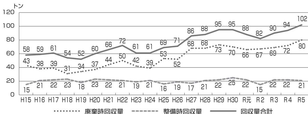
図2-1-6-1 業務用冷凍空調機器からのフロン類回収量の経年変化（2003～2023〔平成15～令和5〕年度）
