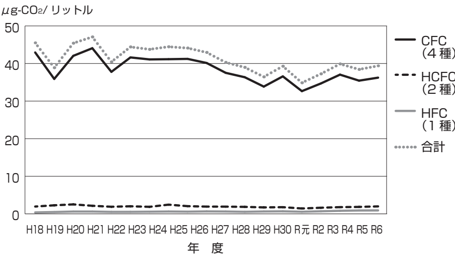
図2-1-6-2 群馬県の大気中における冷媒フロンの経年変化（2006～2024〔平成18～令和6〕年度）
