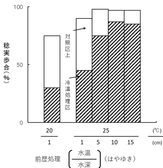
図2 前歴水温上昇による不稔防止効果の水深による差異
