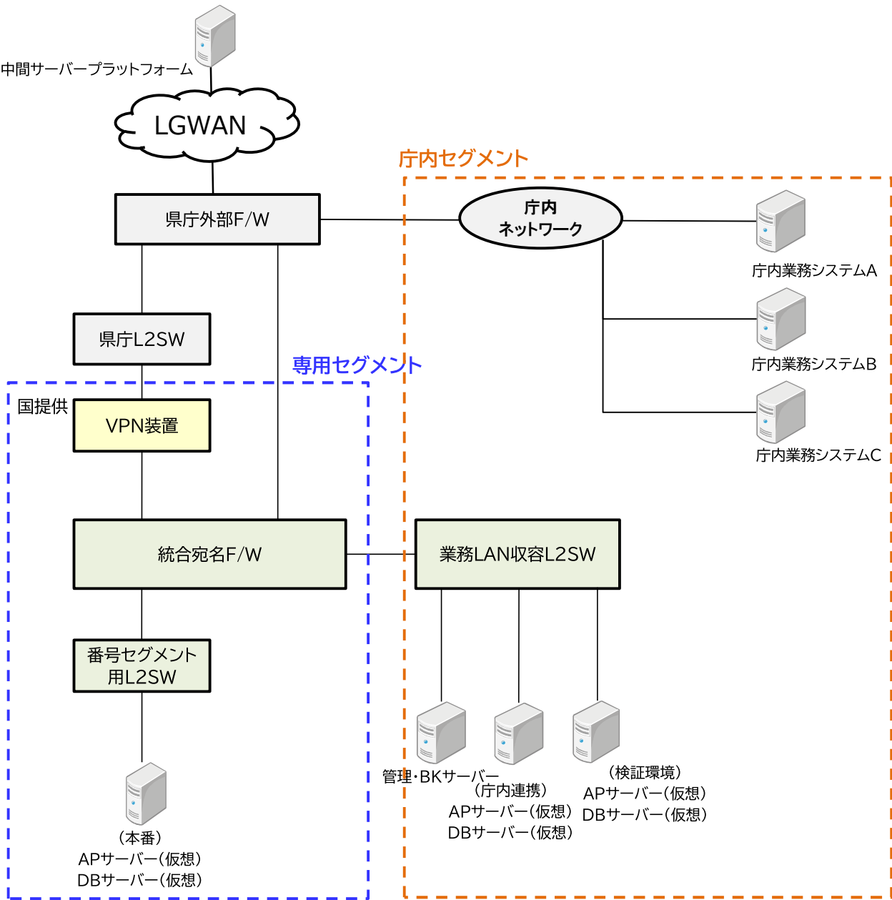
団体内統合利用番号連携サーバ ネットワーク構成図
