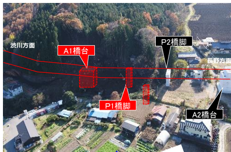
西沢橋 施工状況 (R7.11撮影)
