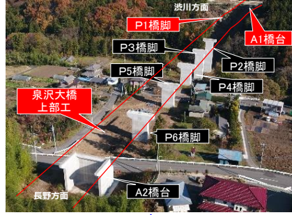
泉沢大橋 施工状況 (R7.11撮影)
