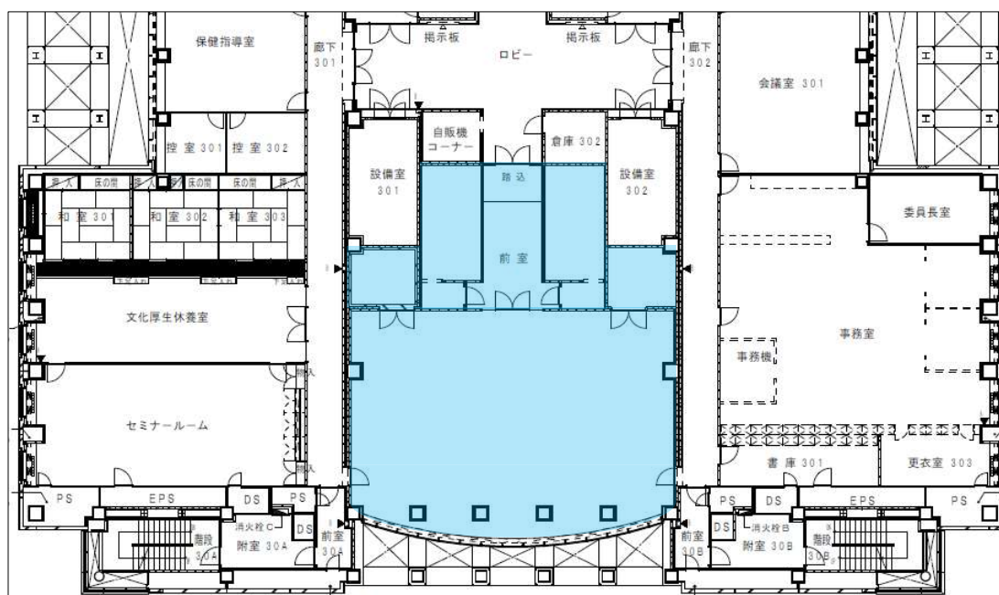
【群馬県庁舎30階図面】
