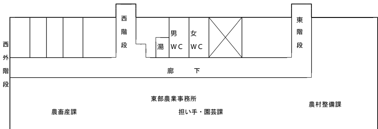
(本庁舎 3 階平面図)
