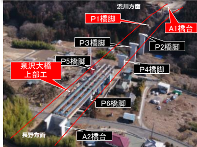
泉沢大橋 施工状況 (R8.2撮影)
