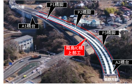
箱島IC橋(渋川方面) 施工状況 (R8.2撮影)
