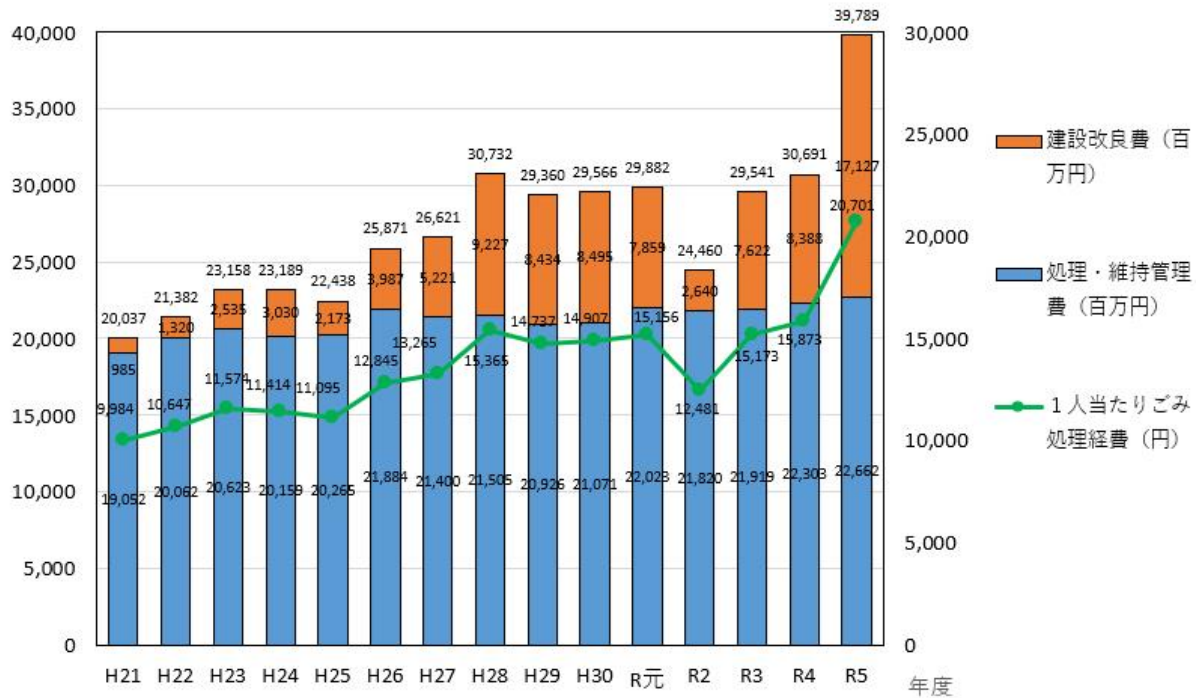
図 2-2-18 ごみ処理経費の推移
