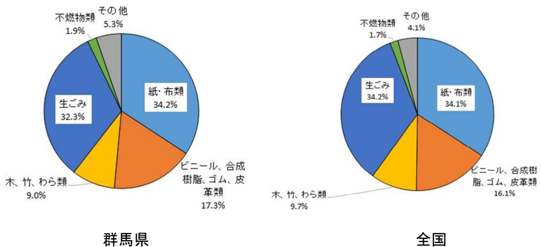
図 2-2-5 焼却施設（溶融施設含む）におけるごみ組成分析結果（湿重量比）（平成 30 年度）
