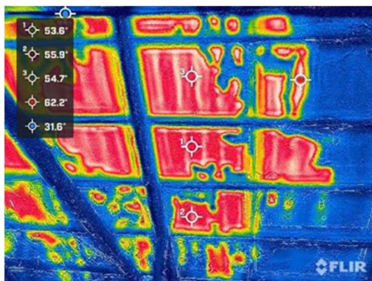
裏面温度
