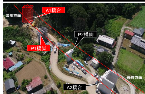
西沢橋 施工状況 (R8. 8撮影)
