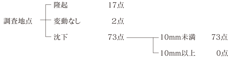
図2-4-1-11 2025（令和7）年度一級水準測量結果
