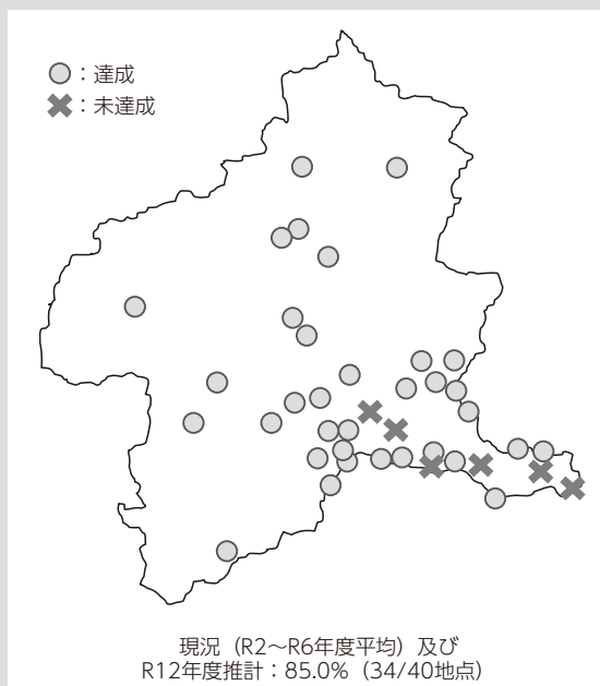
BODの環境基準達成状況
