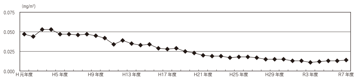
図2-4-2-3 浮遊粒子状物質（SPM）の年平均値経年変化（全測定局平均）
