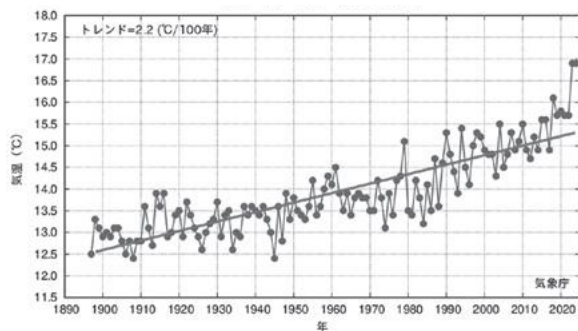
図2-1-2-1 前橋 年平均気温 (1897～2024[明治30～令和6]年)
