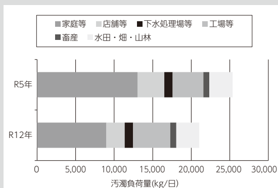
発生源別の汚濁負荷量
