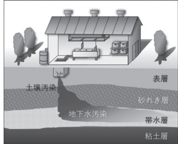
図2-4-1-18 土壌や地下水汚染の模式図
