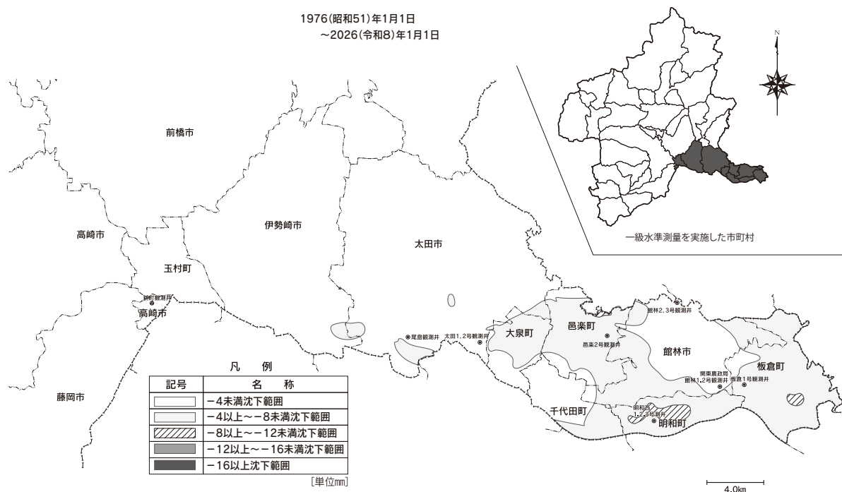
図2-4-1-14 1976（昭和51）年からの年平均地盤変動量図（1976〔昭和51〕年1月1日～2026〔令和8〕年1月1日）
