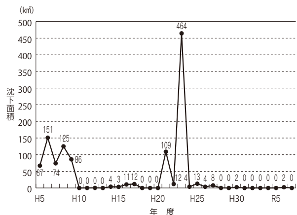
図2-4-1-10 年間10mm以上の地盤沈下面積の推移
