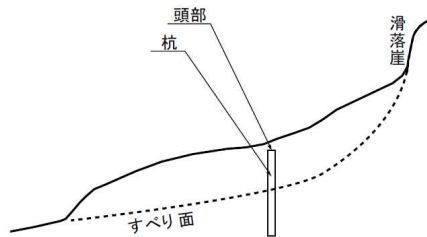
地すべり対策工（杭工）のイメージ
